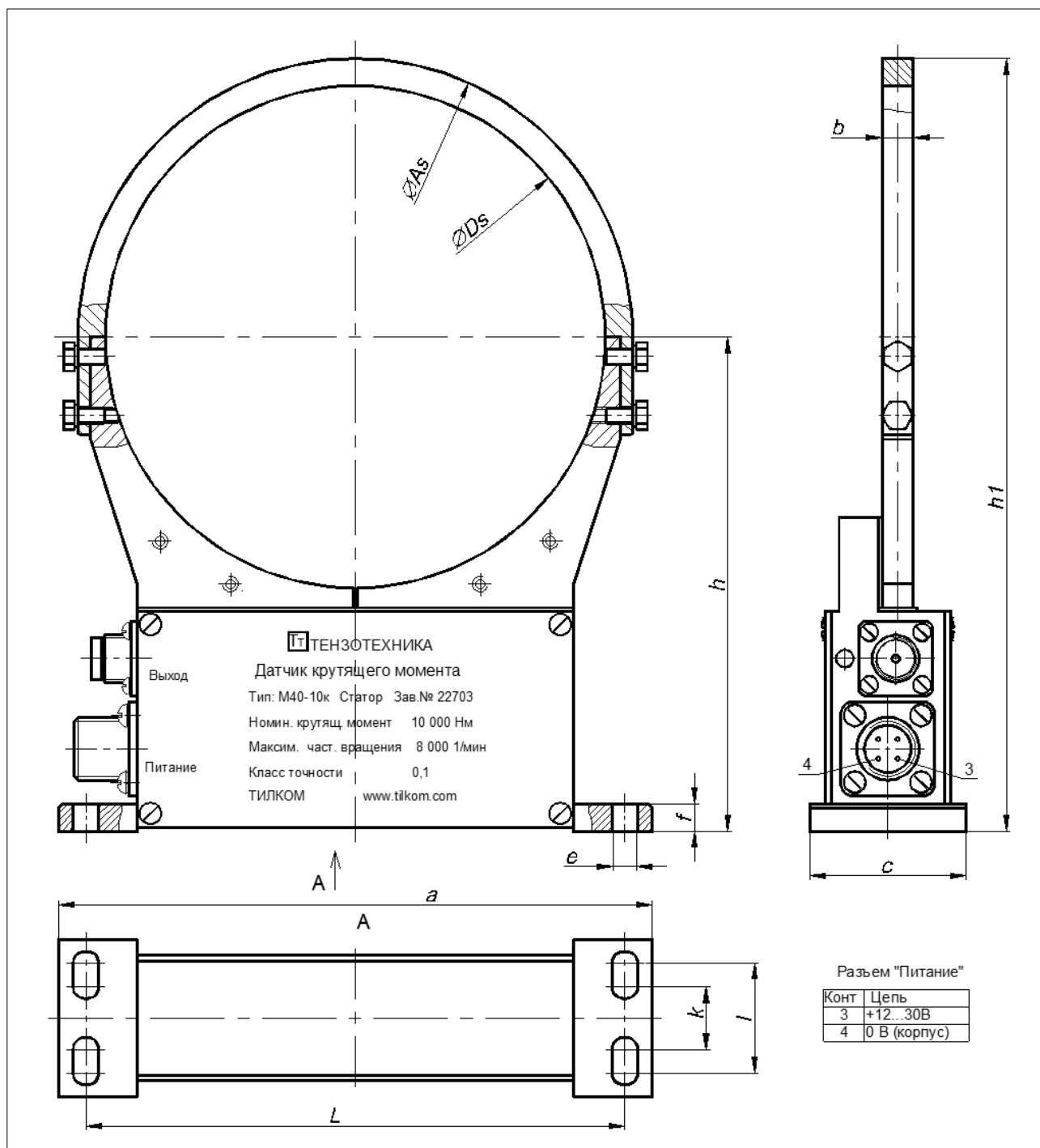
Рис. 8 – Статор М26-3к... М26-5к. Габаритные и установочные размеры, мм
