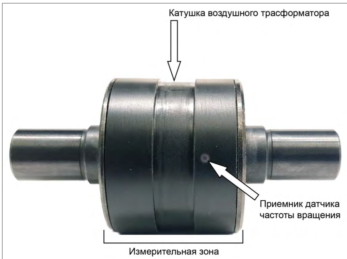
Рис. 2 – Ротор датчика M26
