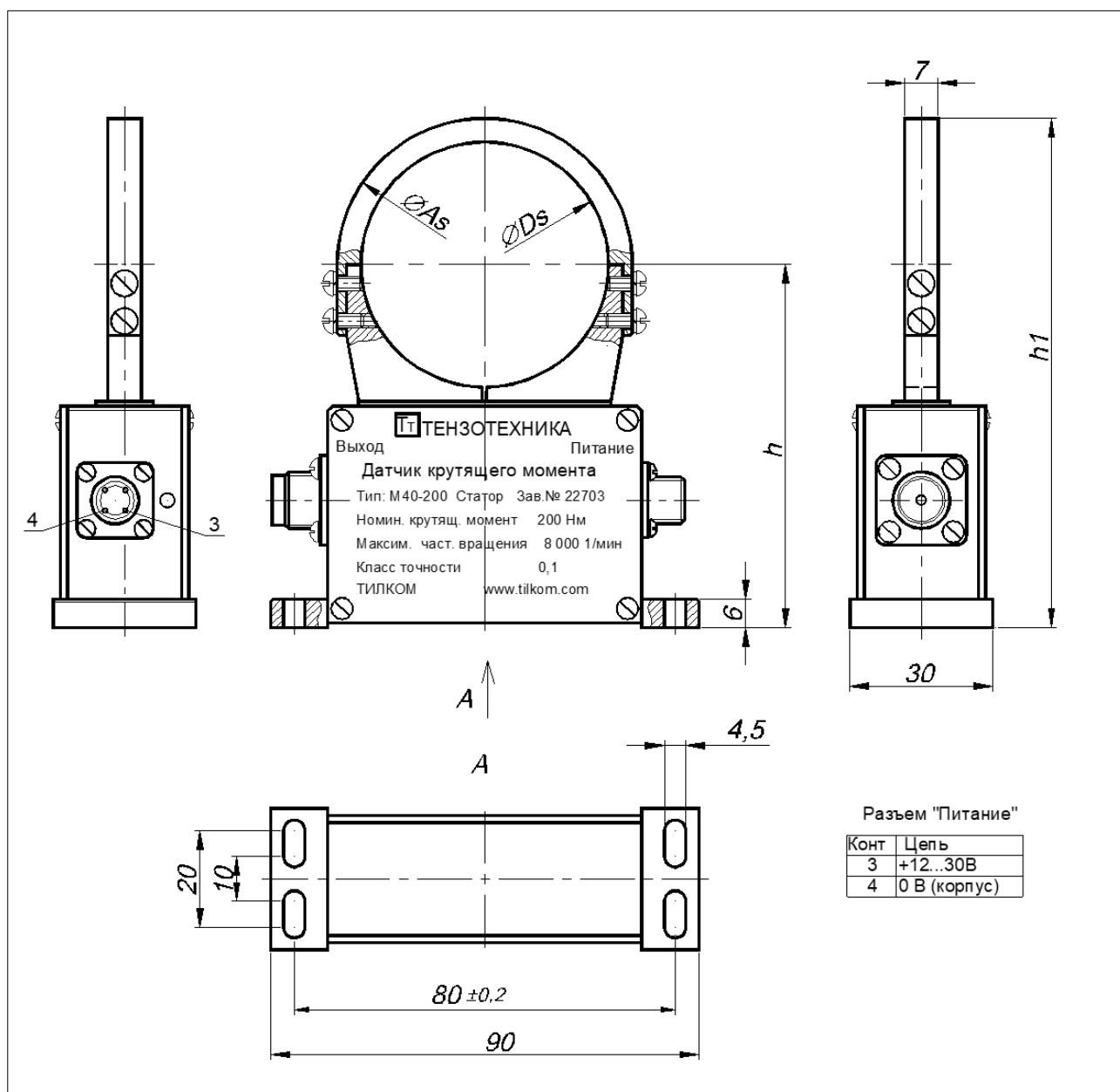
Рис. 6– Статор М26-5... М26-300. Габаритные и установочные размеры, мм
