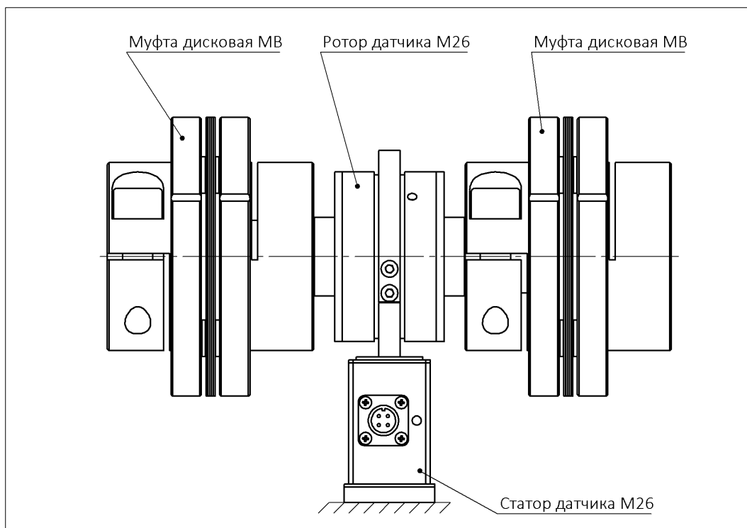
Рис. 9 – Установка датчика M26 с применением дисковых компенсационных муфт MB
