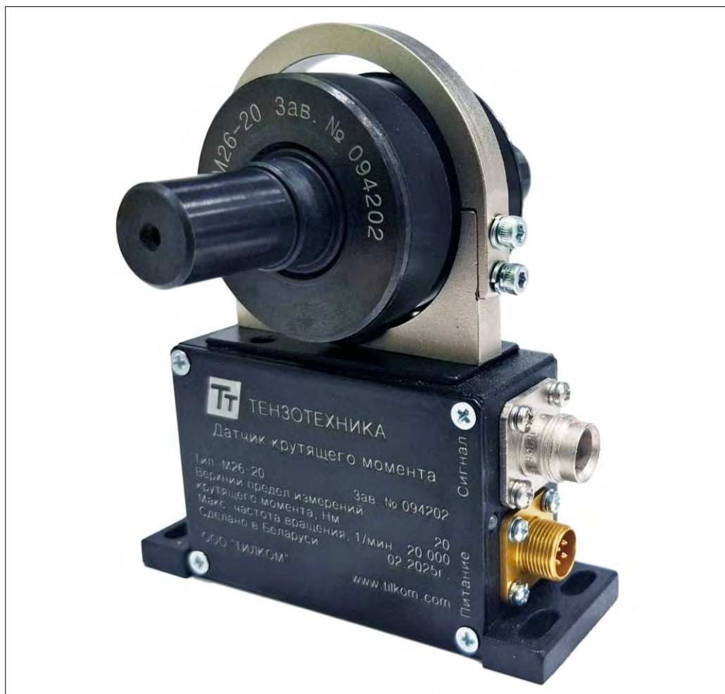
Рис. 1 – Датчик М26
