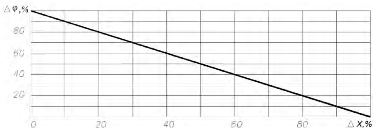
Рис. 10 – Допускаемые сочетания перекоса и осевого смещения компенсационных муфт МК
