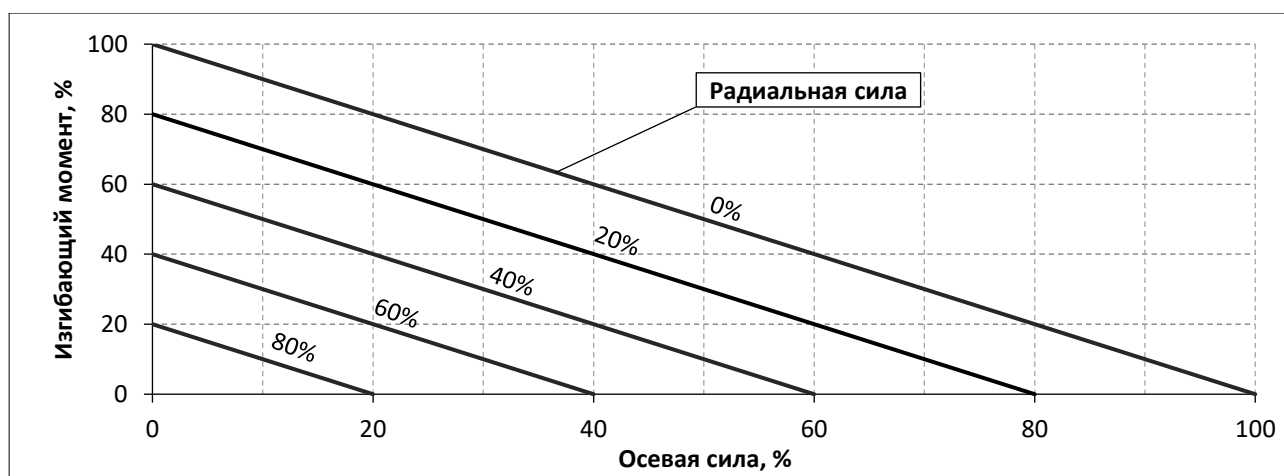
Рис. 4 – Предельно допустимые для датчиков M26 сочетания внешних нагрузок
