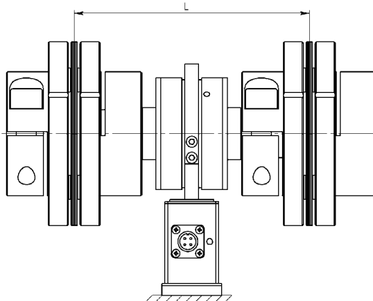
Датчик М26 в сборе с муфтами МВ
