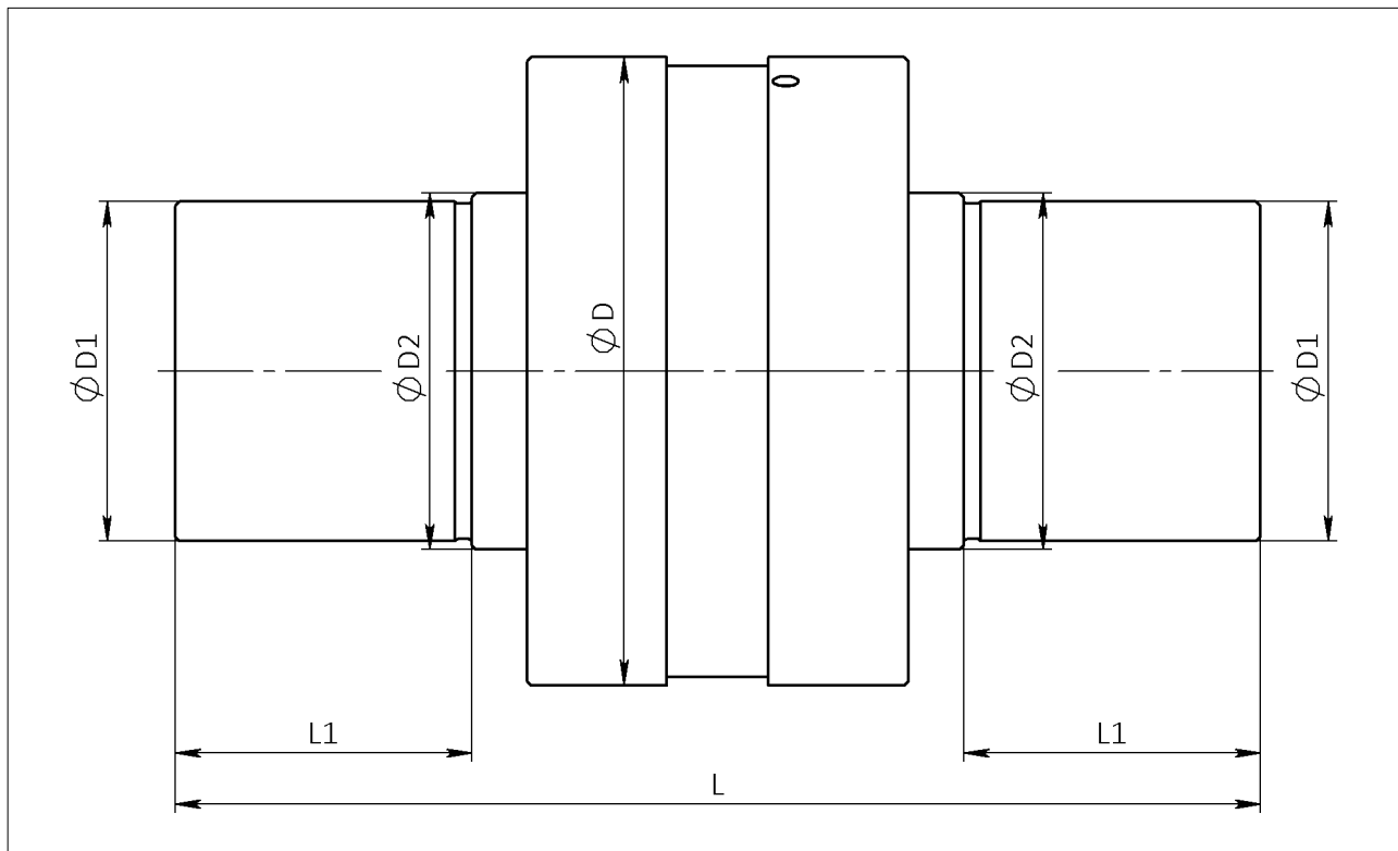
Рис. 5 – Ротор М26. Габаритные и установочные размеры, мм
