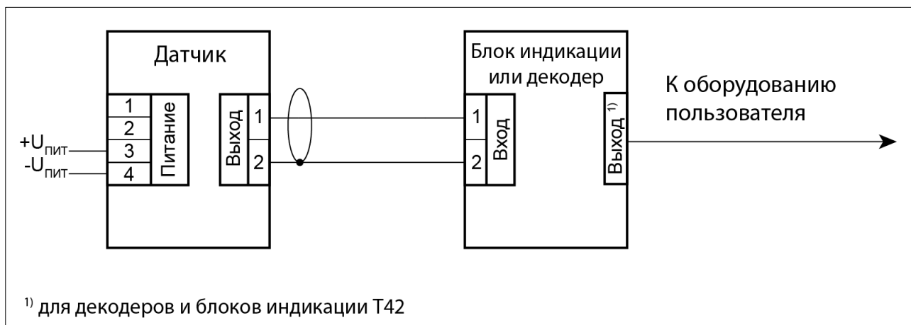
Рис. 13 – Схема подключения датчика M26 к вторичным устройствам
