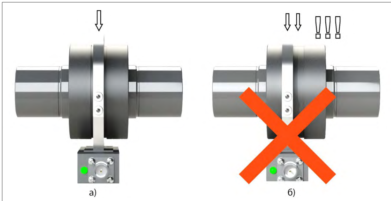
Рис. 11 – Расположение кольца статора относительно катушки ротора: а – ПРАВИЛЬНОЕ, б – НЕПРАВИЛЬНОЕ
